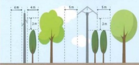
LIGNES HAUTE TENSION (HTA) - 15 ou 20 000 volts Attention : les distances varient selon les types de lignes.
